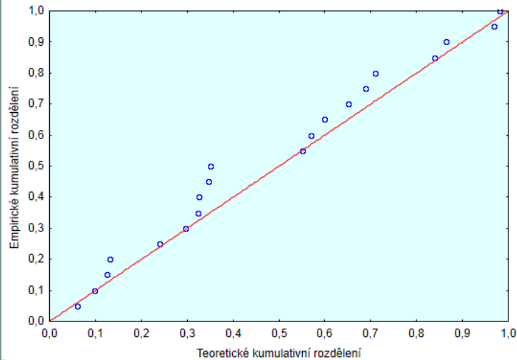
Graf P-P
