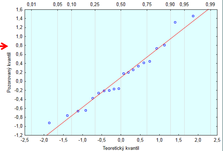
Graf Q-Q
