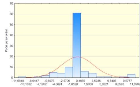
Špičatost
