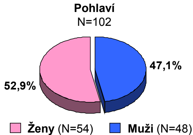
Koláčový graf
