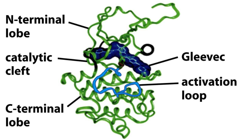
Model kinázy Abl
