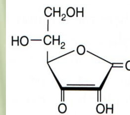
Monodehydroaskorbát (semidehydroaskorbát)
