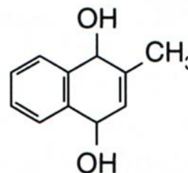
Menadiol
