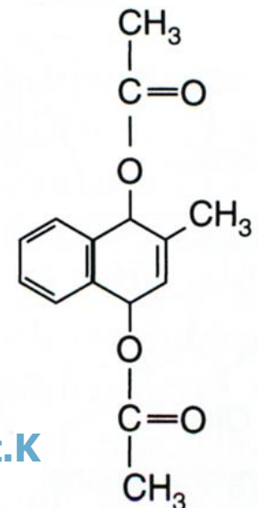
Menadiol diacetát
