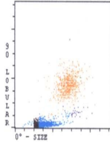
Optical PLT
