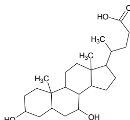
Kyselina chenodeoxycholová
