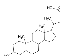
Kyselina lithocholová
