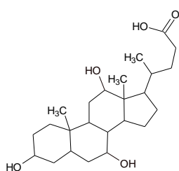
Kyselina cholová
