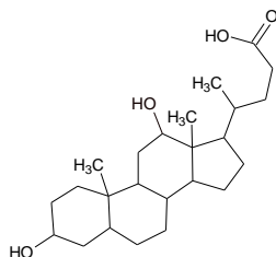
Kyselina deoxycholová
