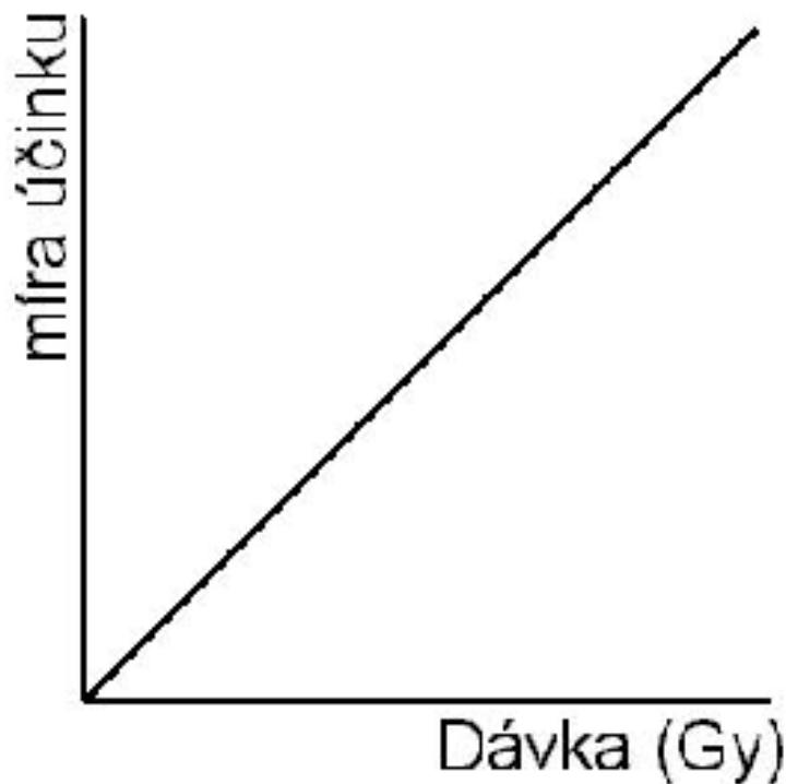
účinky stochastické
