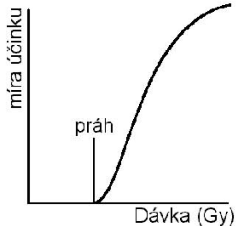
účinky deterministické
