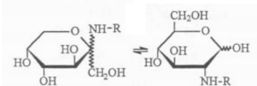
D-fruktosylamin
