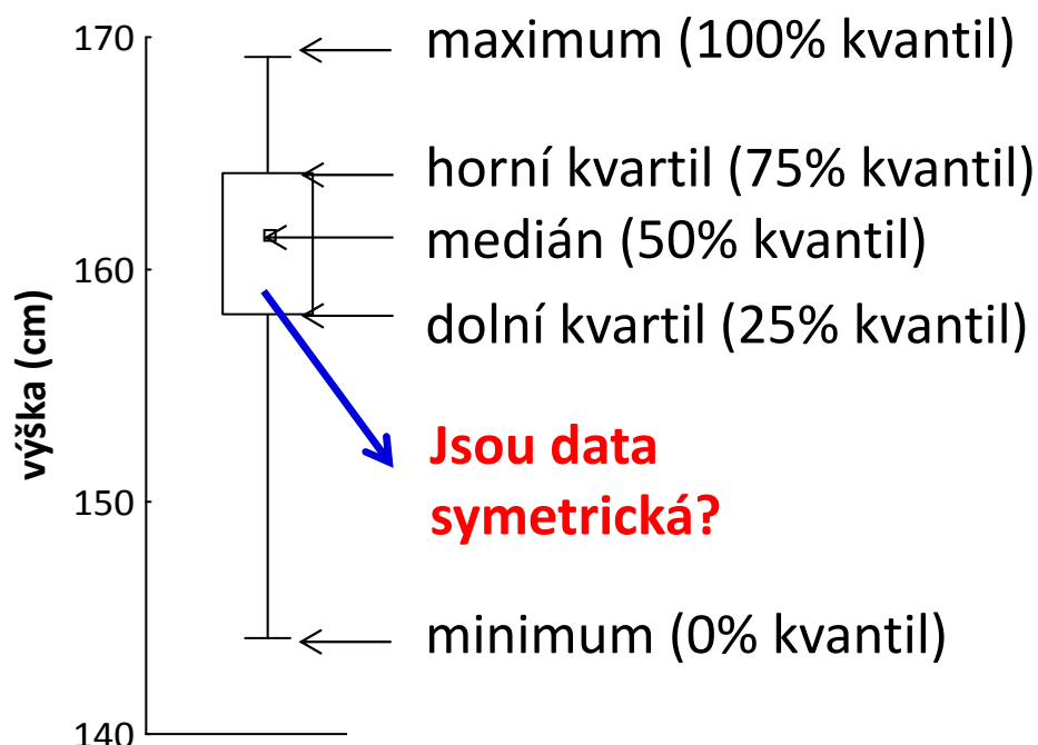
Krabicový graf
