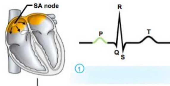
Depolarizace síní
