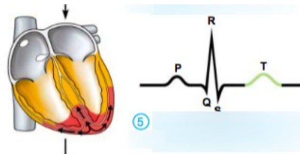
Repolarizace komor
