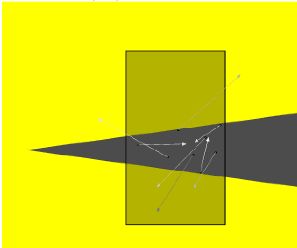
Obrázek 3.1.1 Comptonův jev. Paprsek prozařuje hranol a z ozářené části vyletují náhodně smerované comptonovské fotony.
