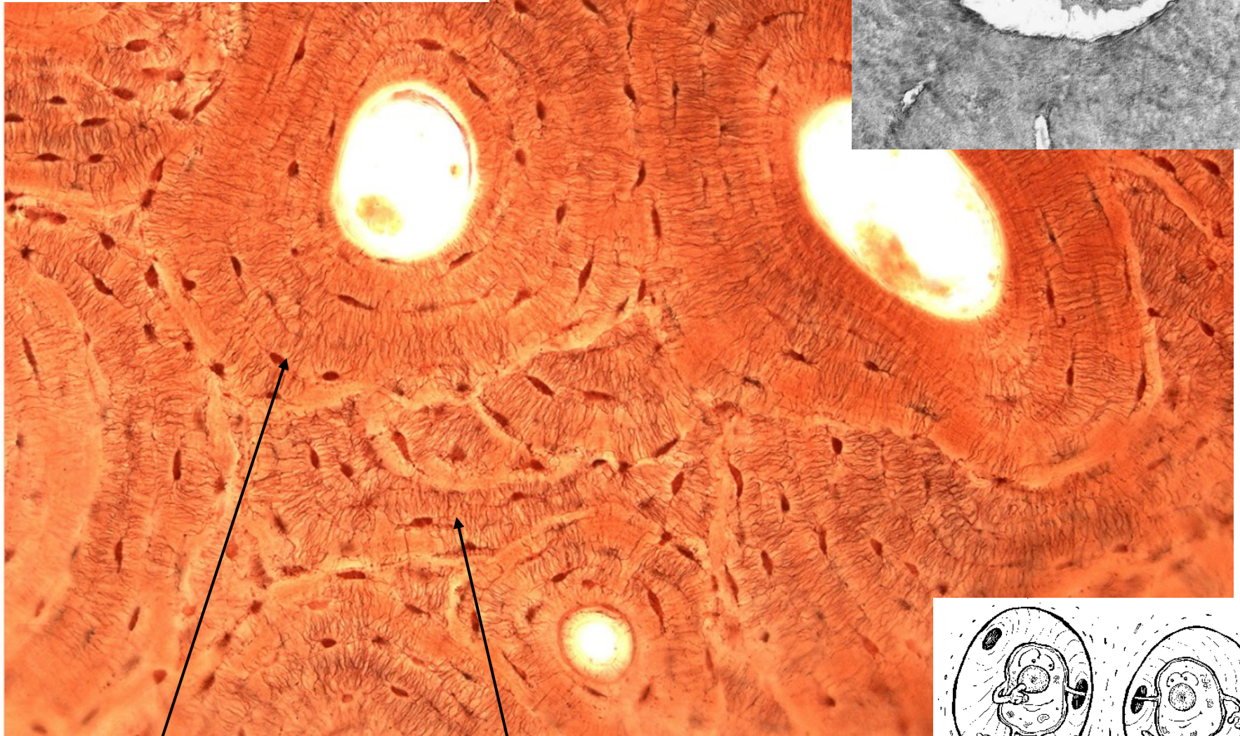
Kompletní osteon
