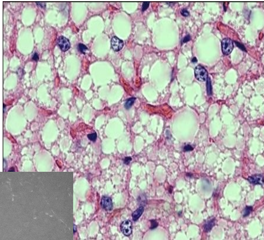
multivakuolární
