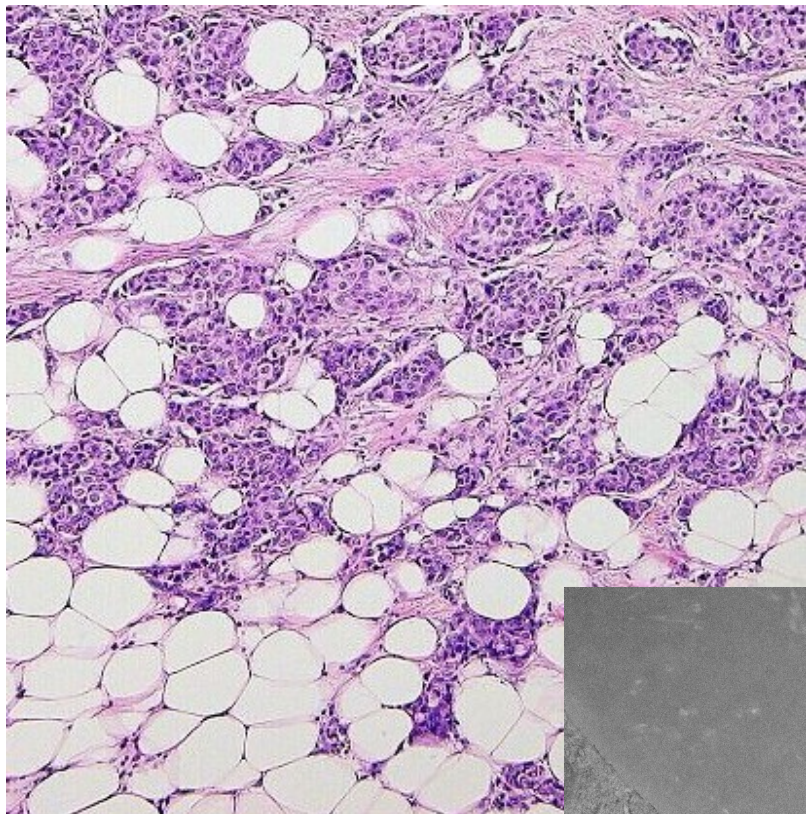
univakuolární
