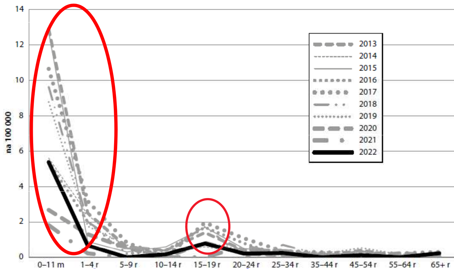
Graf 4: Invazivní meningokokové onemocnění – specifická věková nemocnost. Česká republika, 2013–2022, surveillance data
