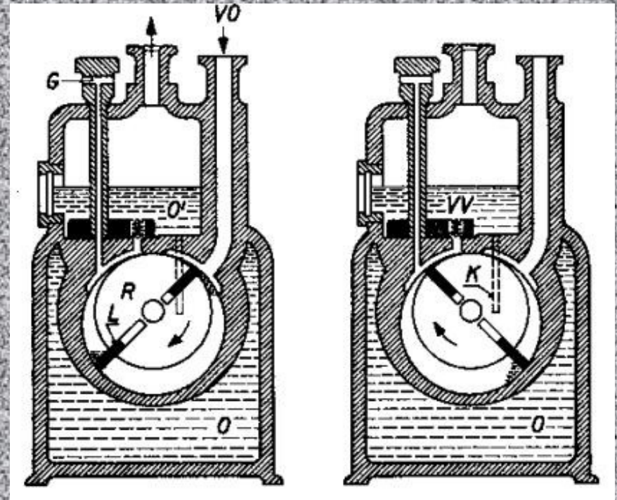
Oleřová rotační vývěva
