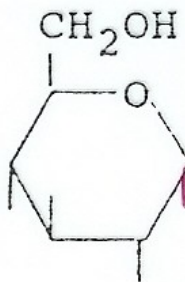
\alpha -glucopyranose
