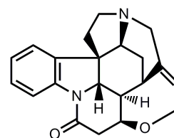
strychnine
