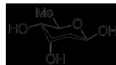
digitoxose
