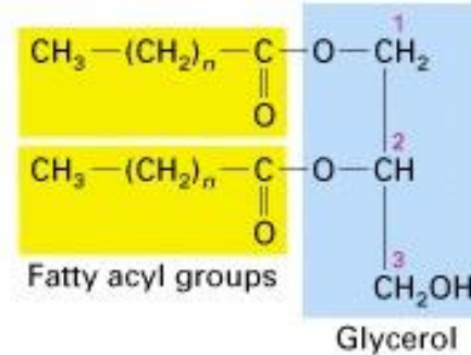
1,2-Diacylglycerol (DAG)
