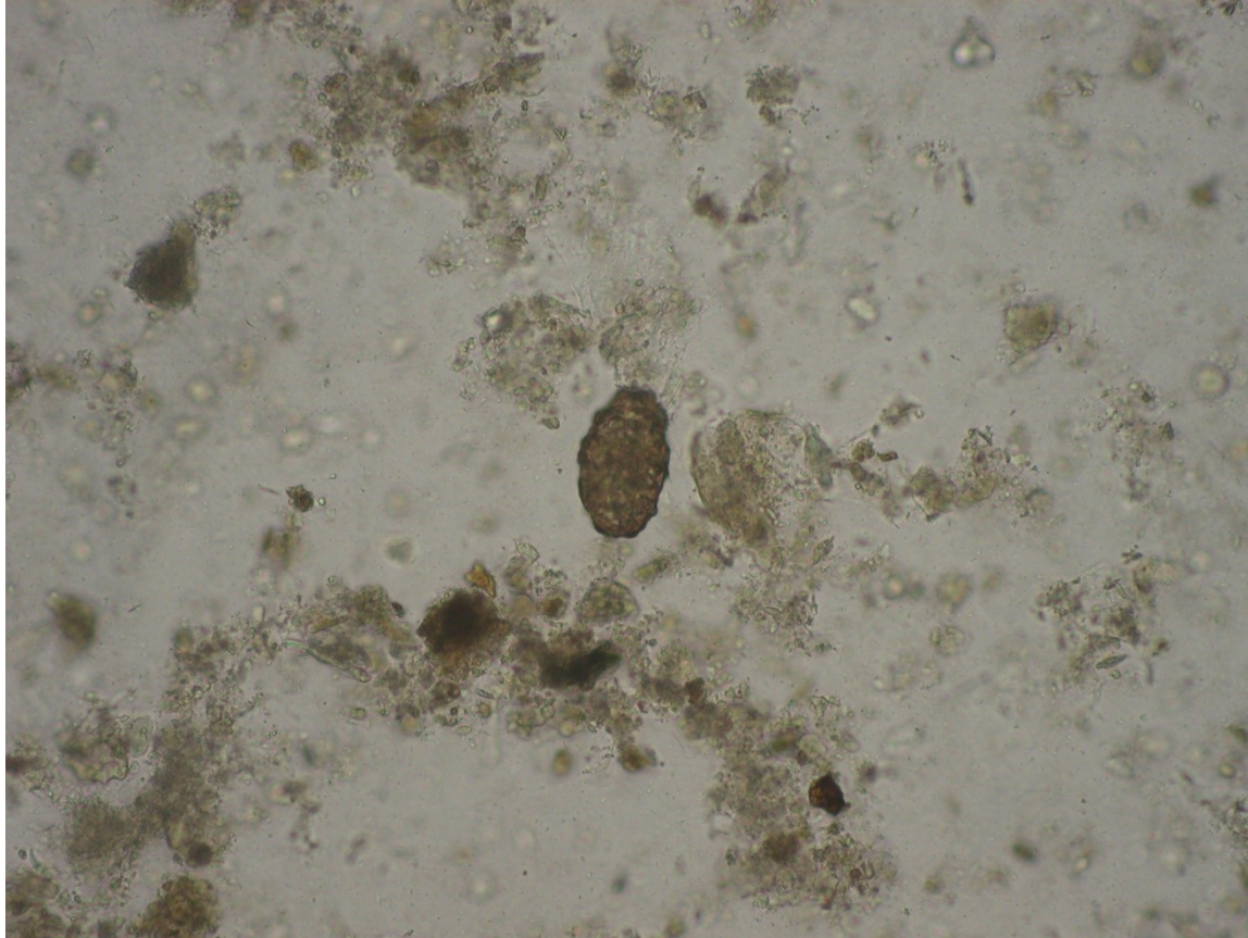
Ascaris lumbricoides - egg
