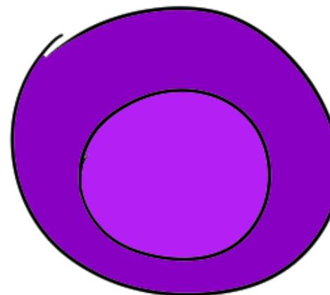
Myelomová buňka
