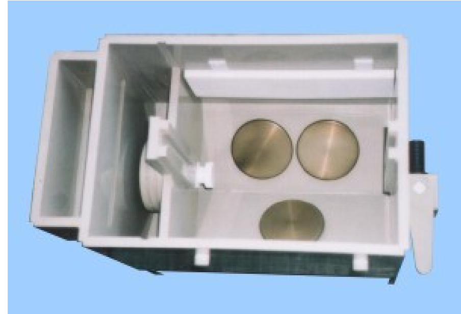
Ultrazvuková lázeň - pohled shora (okrouhlé destičky jsou zdroje ultrazvuku)
