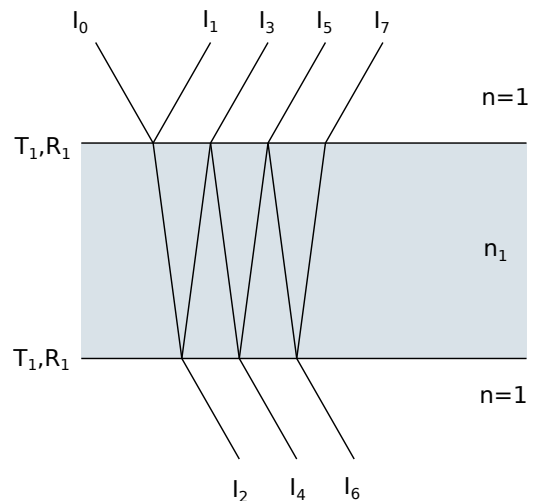
Obr. 1: Planparalelní deska ponořená do vzduchu.
