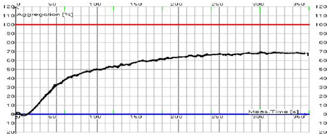
ADP 5 \mu\text{M} desagregace – křivka č. 6
