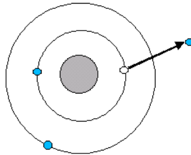
ionizace
