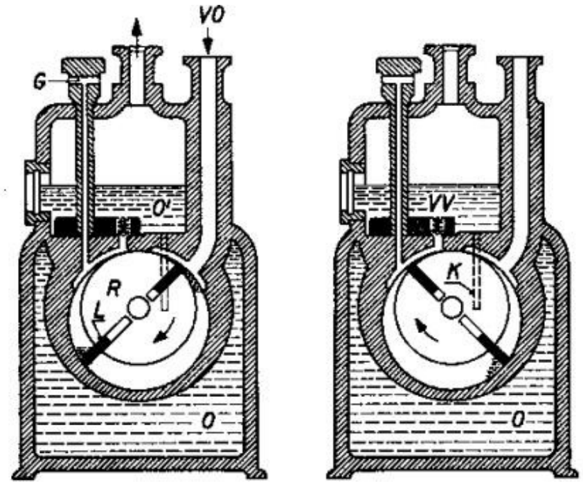
Olejevá rotační vývěva
