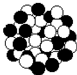
Mn 55
