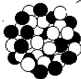
Fe 55
