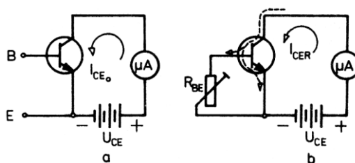
Obr. 1.13 Zbytkový proud tranzistoru. (Převzato z [1]).
