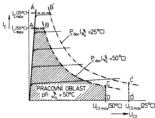
Obr. 1.18 Pracovní oblast tranzistoru. Při \vartheta_a = +50^\circ\text{C} omezena body ABCDO, při teplotě \vartheta_a = +35^\circ\text{C} omezena body A'B'C'D'O. (Převzato z [1]).
