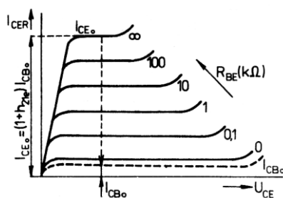
Obr. 1.14 Vliv odporu mezi bází a editorem na zbytkový proud tranzistoru. (Převzato z [1]).
