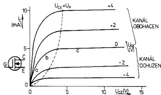
Obr. 1.7 Výstupní charakteristiky tranzistoru MISFE s vodivým kanálem. (Převzato z [1]).
