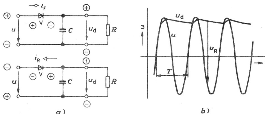
Obr. 1.4 a) Jednopolusní usměrňovač zatížený na výstupu paralelní kombinací odporu a kapacity, b) časový průběh napětí u_d . (Převzato z [15]).
