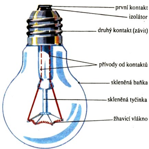
Obr.4.42. Žárovka
