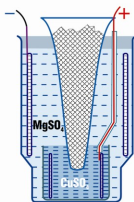
Obr.1.7b) Meidingerův článek
