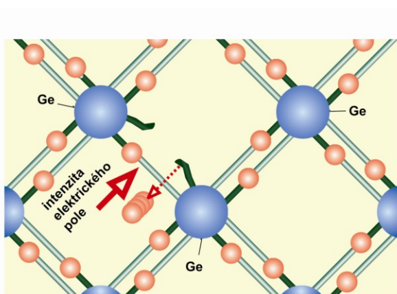
Obr.3.3. Elektronová vodivost v polovodičích
