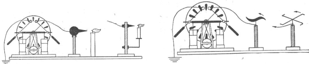
Obr. 5.5. Důkaz sršení náboje z hrotu.
