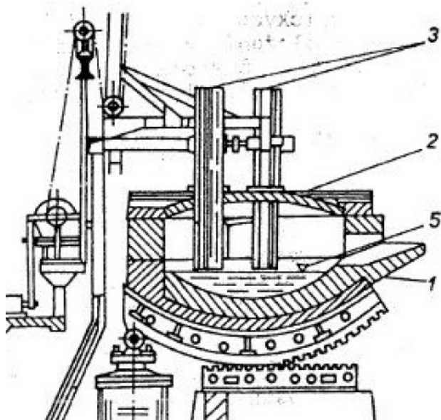
Oblouková pec
