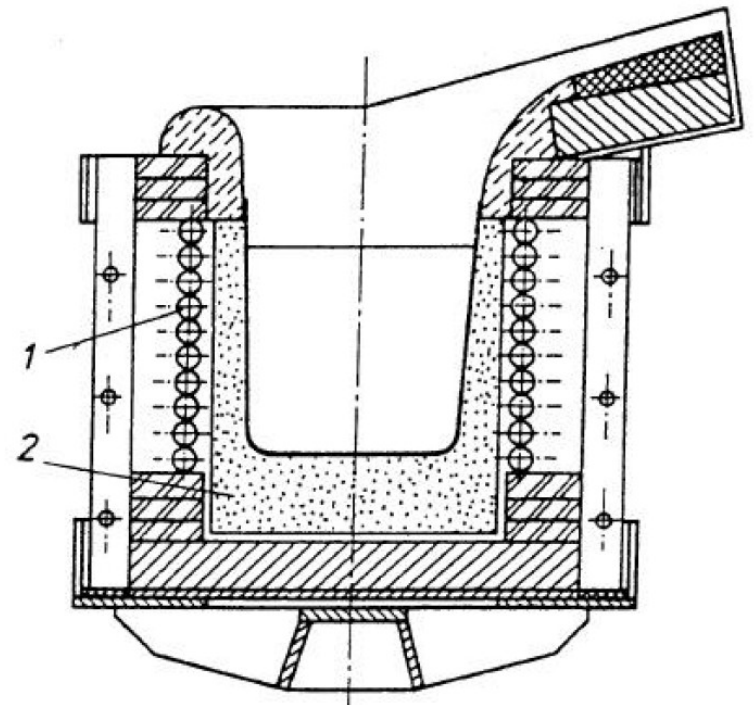
Indukční pec
