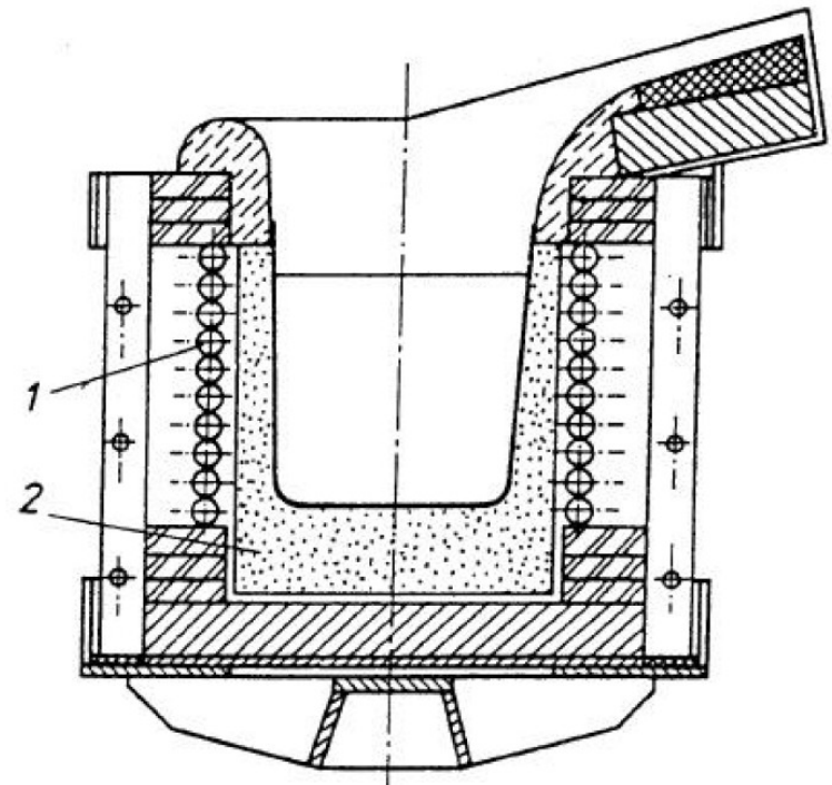
Indukční pec
