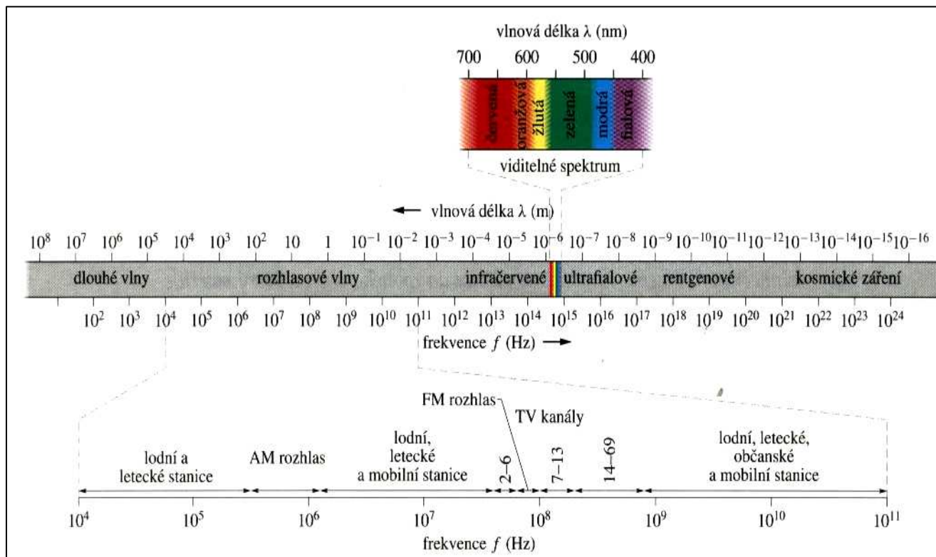
Obr.1. Elektromagnetické spektrum
