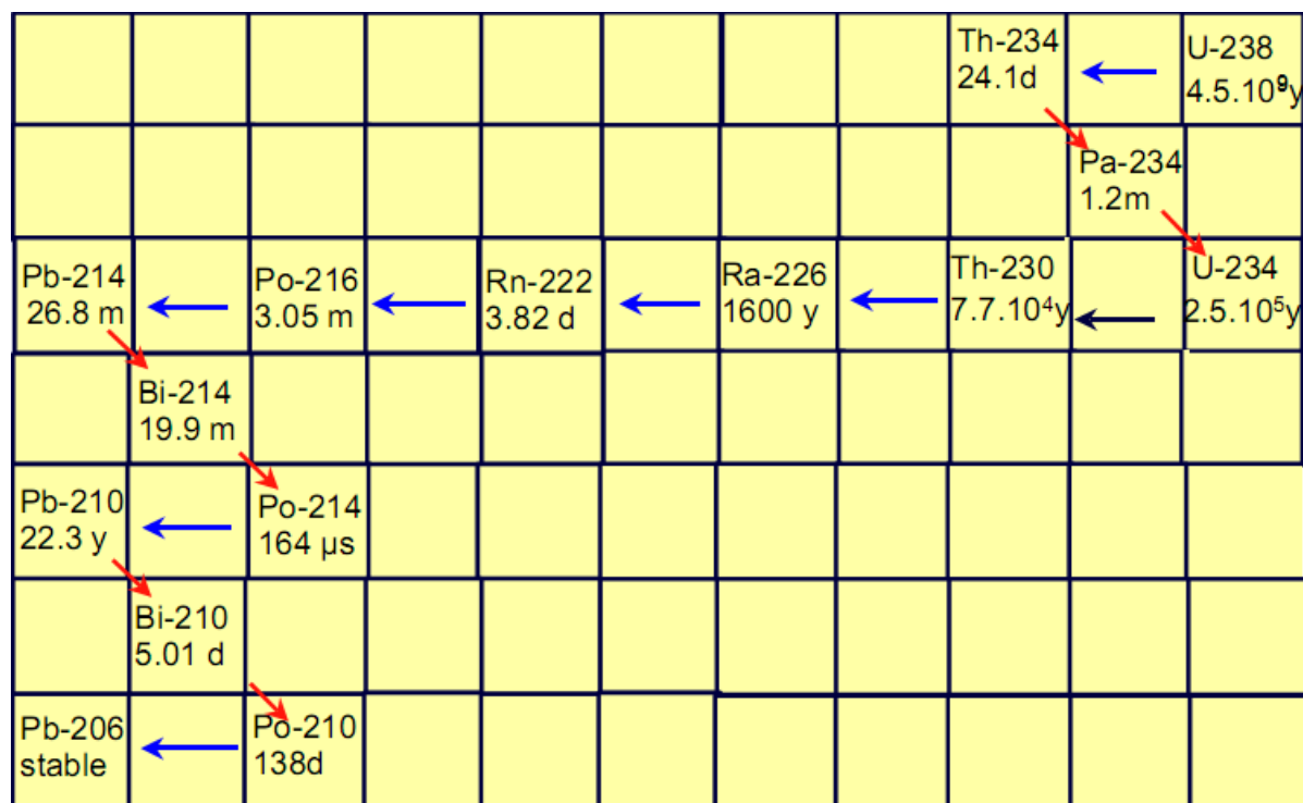
Obr.14. Rozpadová řada ^{238}\text{U} a dceřinné produkty radonu.
