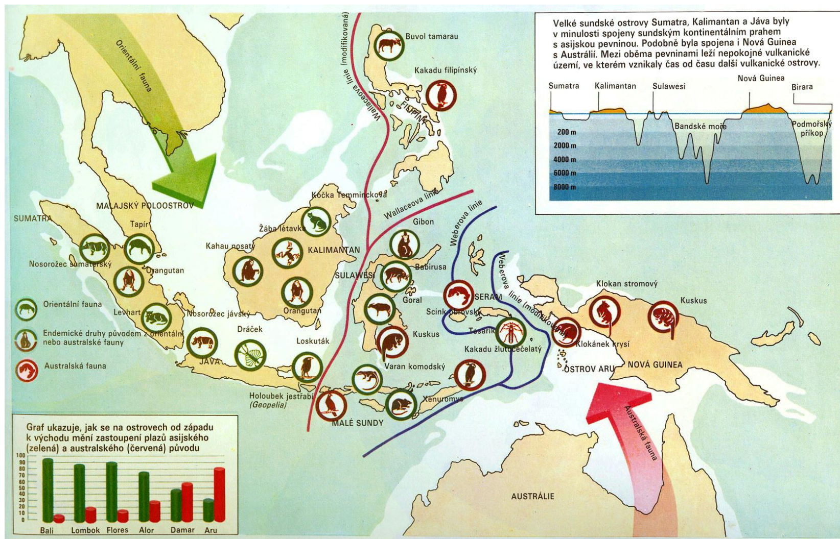
Obr. 42: Variabilita navržených hranic indomalajské a australasijské biogeografické oblasti (Kol., 2005) – podrobnější vyjádření
