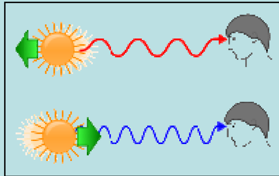
Rudý a modrý posuv spektrálních čar
