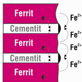
Obr.1.10. Strukturní korozní dvojice ferrit – cementit.
