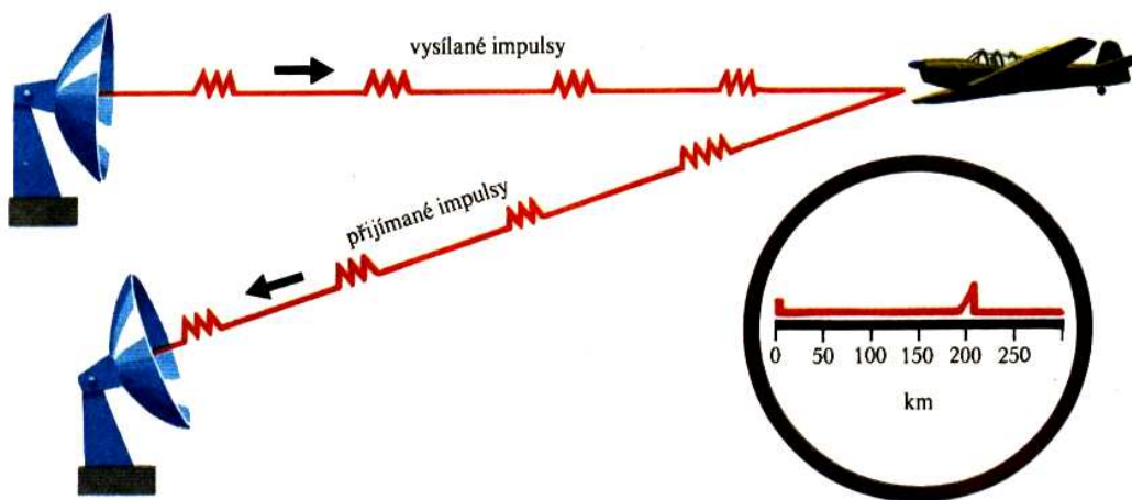
Obr.4.56. Princip činnosti radaru.
