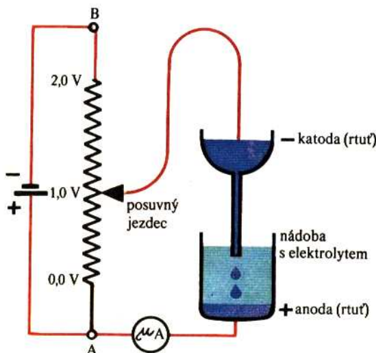
Obr.4.26. Polarograf
