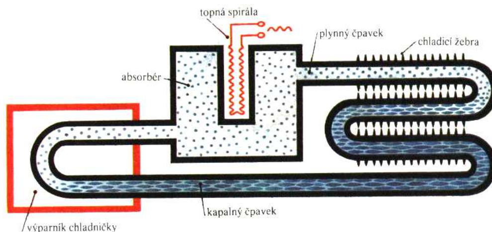
Obr.4.3. Princip absorbční chladničky.
