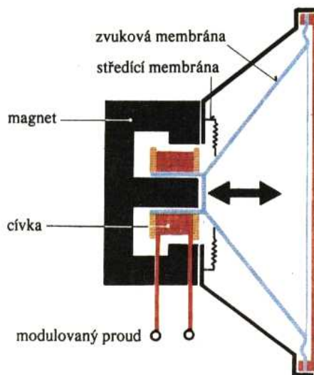
Obr.4.61. Elektromagnetický reproduktor.
