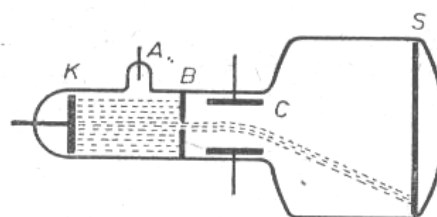
Obr.5.30. Vychýlení katodových paprsků elektrickým polem.
