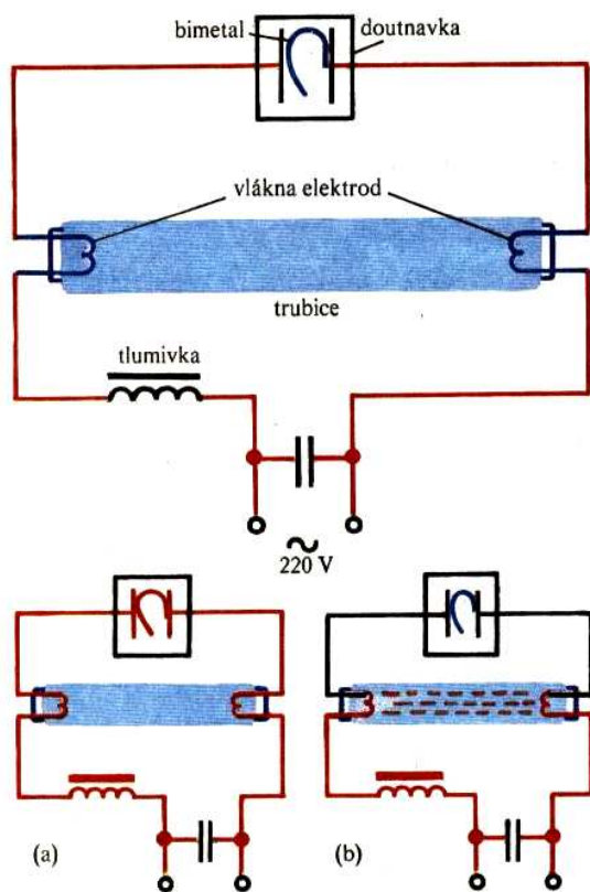
Obr.4.45. Zářivka
