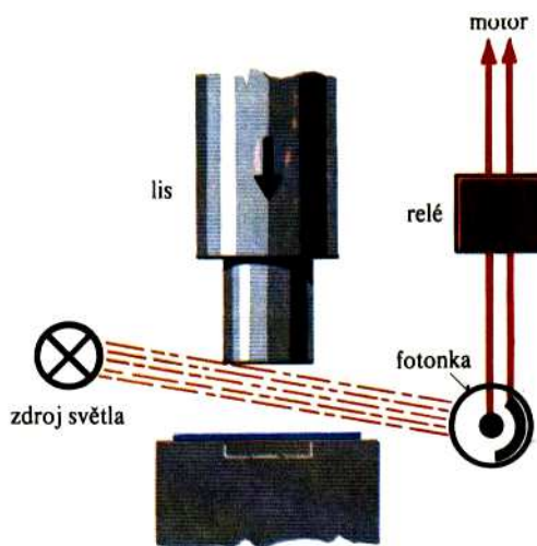
4.51. Jedno z možných využití fotonky v praxi.
