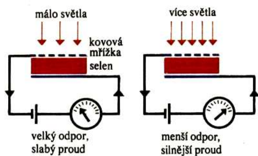
Obr.4.47. Vnitřní fotoefekt
