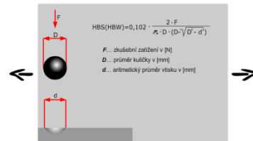
Vztah pro výpočet tvrdosti podle Brinella
