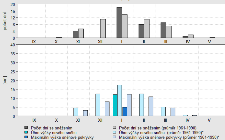
Měsíční charakteristiky sněhu pro zimní sezónu 2015/2016 ve srovnání s dlouhodobým průměrem 1961-1990
