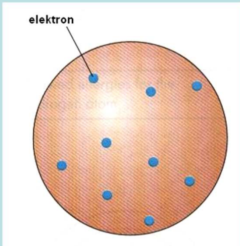
Pudinkový model
