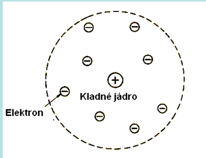
Rutherfordův model
