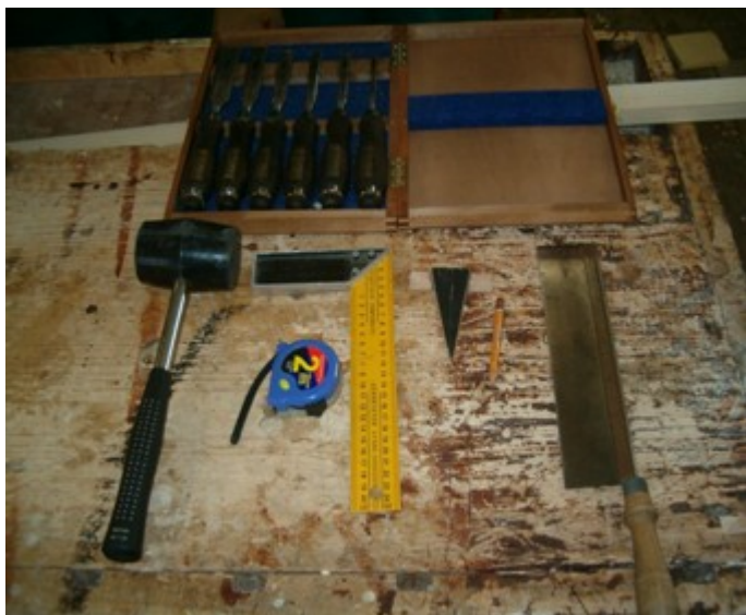
Obrázek č. 4: Vybrané ruční nástroje pro cvičnou práci v oboru truhlář - zhotovení čepového spoje (Kovář, 2011, s. 51)
