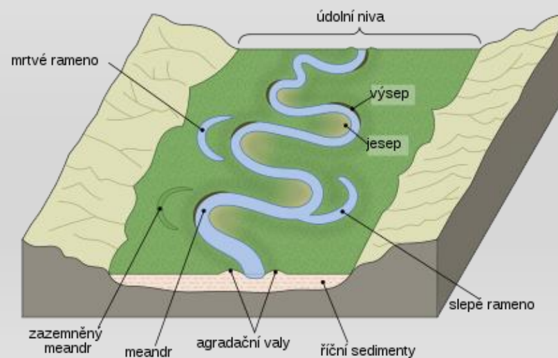
Profil fluviálními sedimenty.
