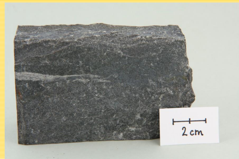
Masivní, jemně zrnitá stavba kontaktního rohovce, Bělce u Neveklova.
