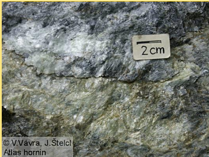
Mastková břidlice, Zadní Hutisko.
