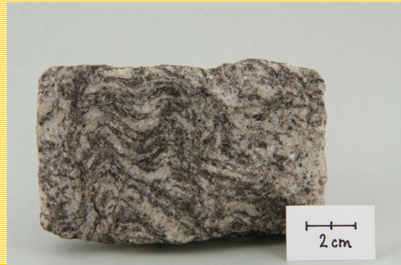
Jemně provrásněná migmatitizovaná rula, Tábor.
