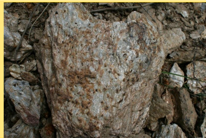
Porfýroblasty granátu ve svoru s výraznou foliací, Sobotín.
