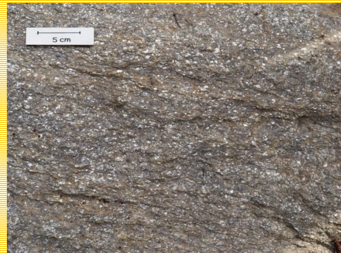
Tabulky muskovitu na plochách foliace svoru, Oslavany.
