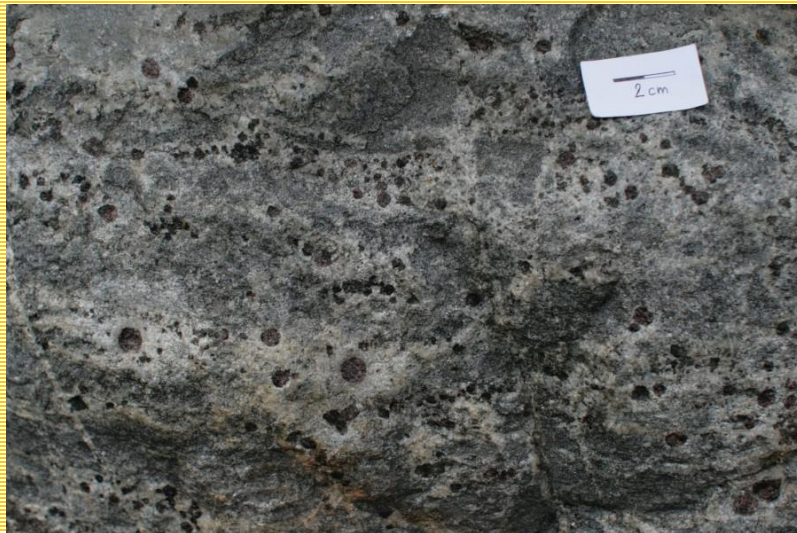
Migmatitizovaná tula s porfiroblasty granátu, Tábor.
