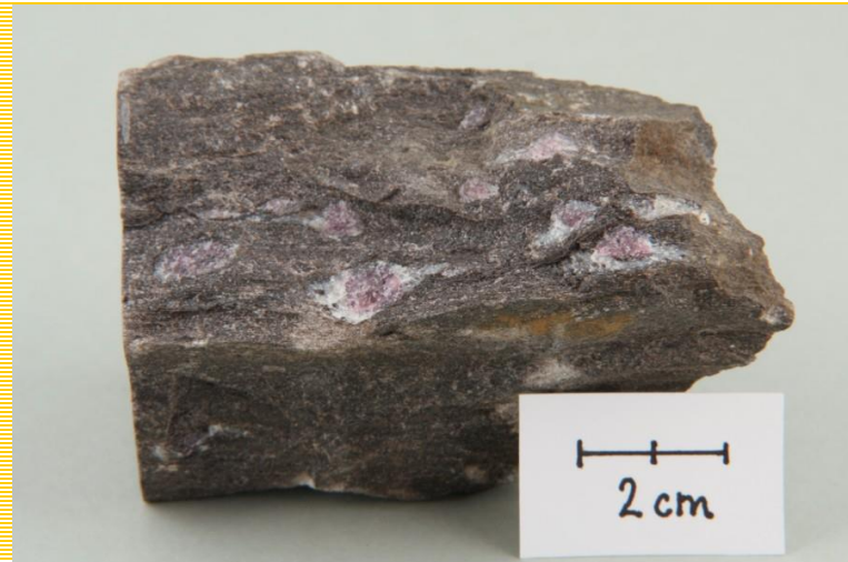
Rula s porfyroblasty granátu, Starkoč.
