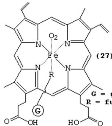
Oxyhaemoglobin
