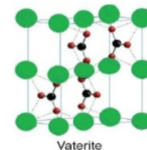
Vaterite
