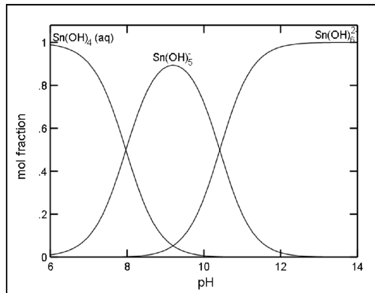
Speciační diagram pro Sn(IV)
