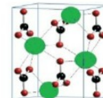
Aragonite
