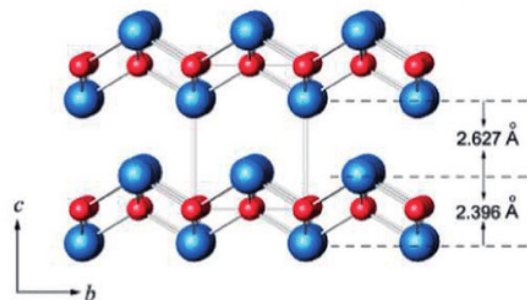
\alpha -PbO:
