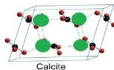
Calcite
