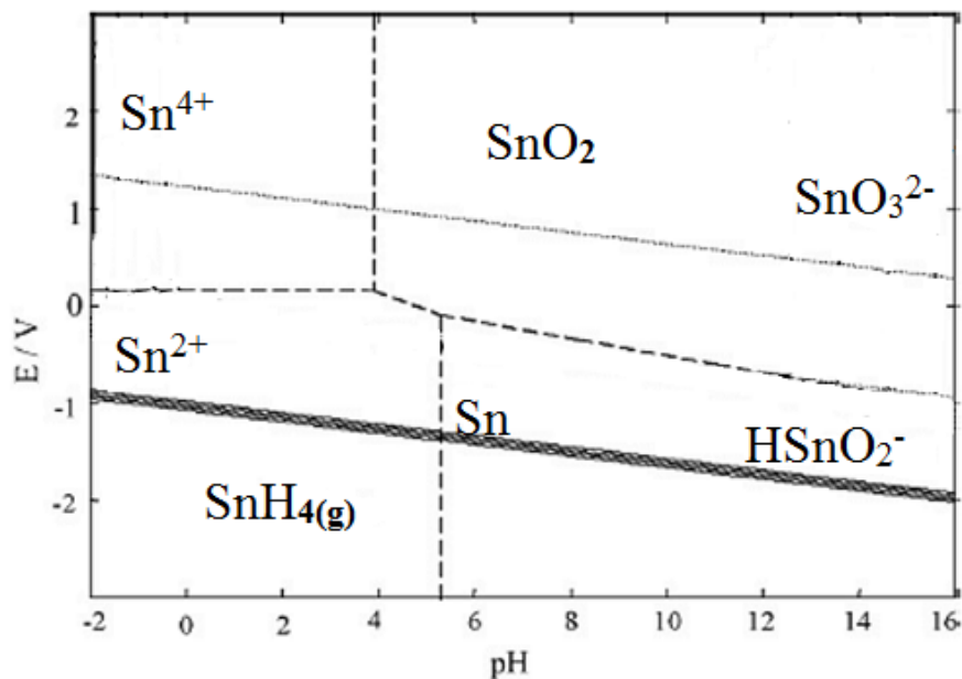
Pourbaixův diagram pro Sn
