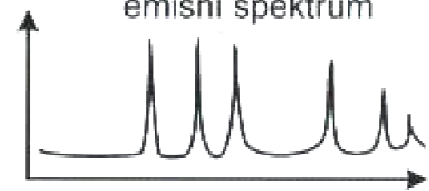
emisní spektrum
