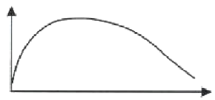
spojité spektrum
