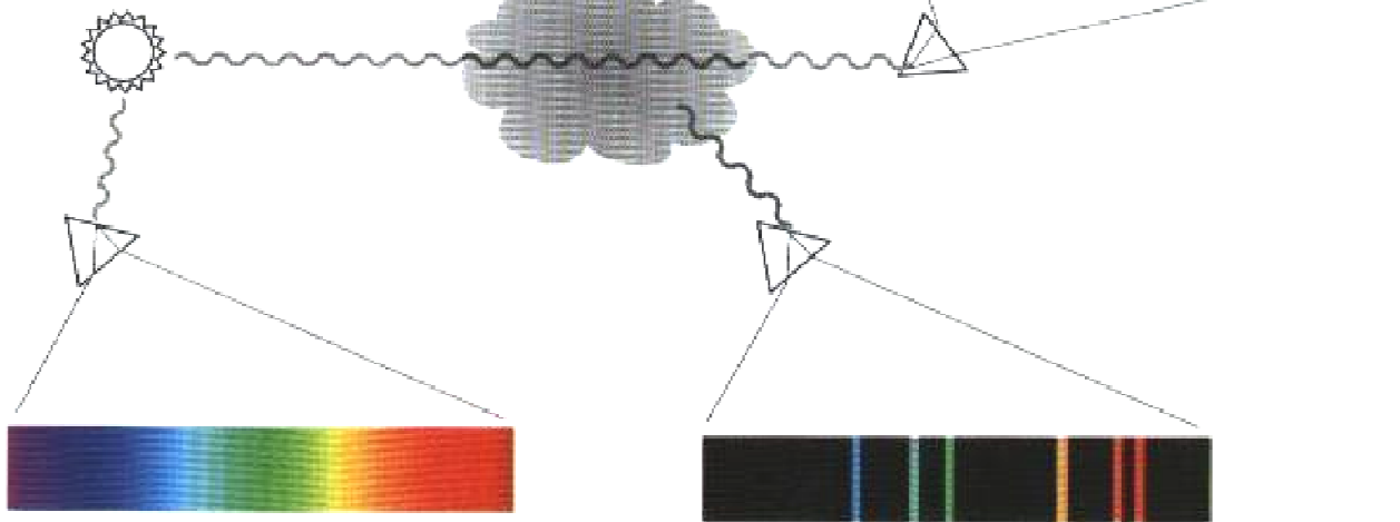
spojité spektrum
