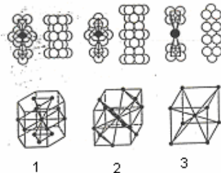
Obr. 65: krystalické struktury kovů: a – model struktury, b – krystalové mřížky; 1 – šesterečná, 2 – krychlová plošně centrovaná, 3 – krychlová tělesně centrovaná
