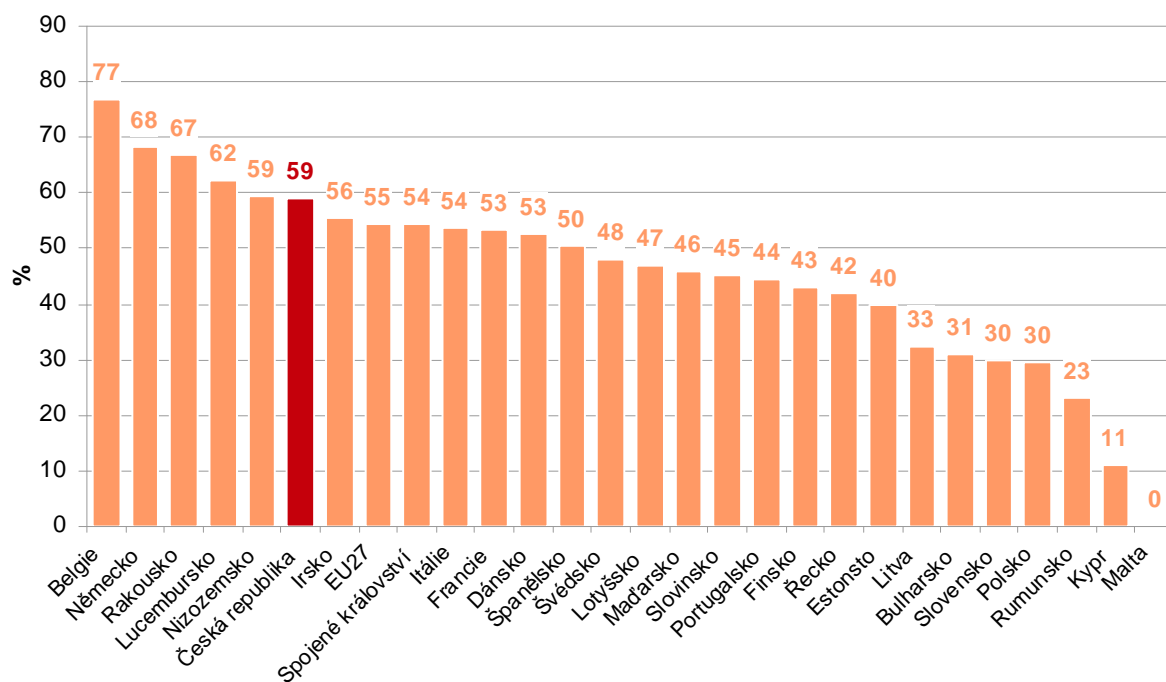
Graf 3 Míra recyklace a využití obalového odpadu v roce 2007
