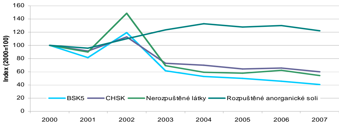
Graf 1 Vypouštěné znečištění v letech 2000–2007
