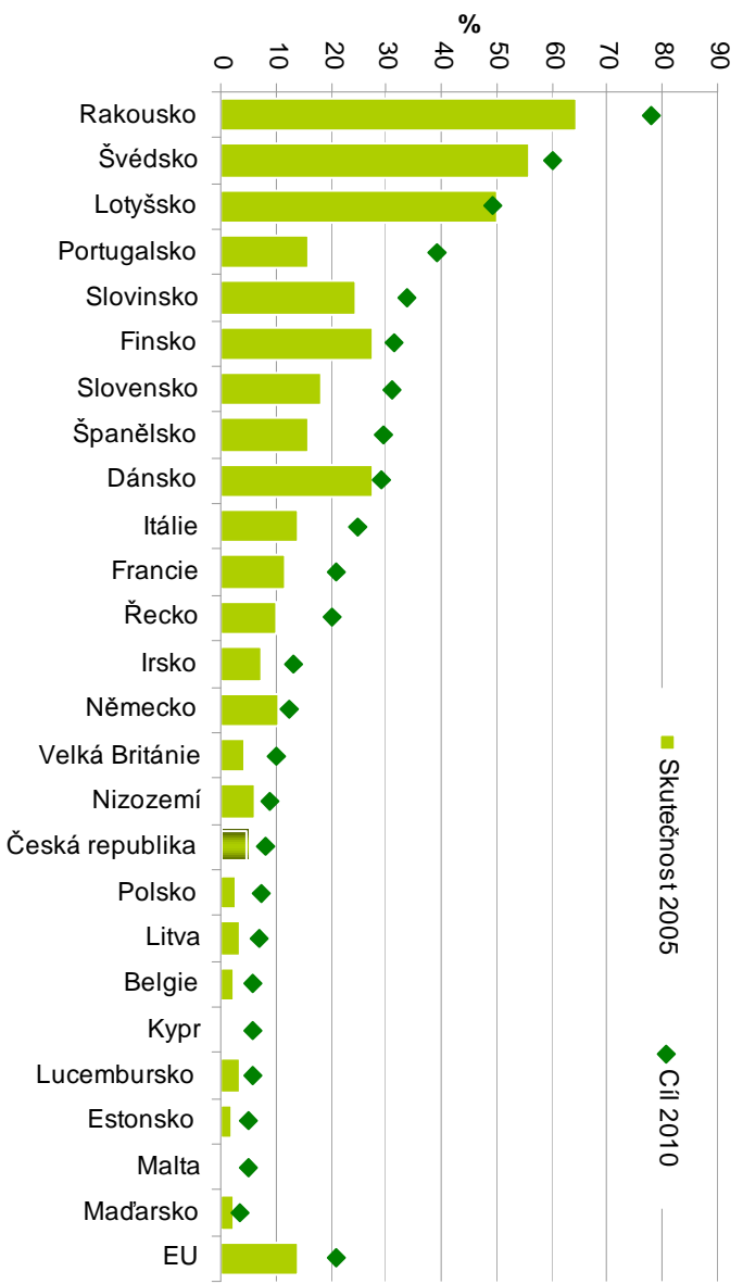
Graf 3 Mezinárodní srovnání využívání OZE na hrubé spotřebě elektřiny
