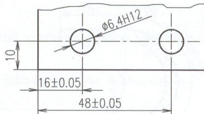
Technologické kótování
