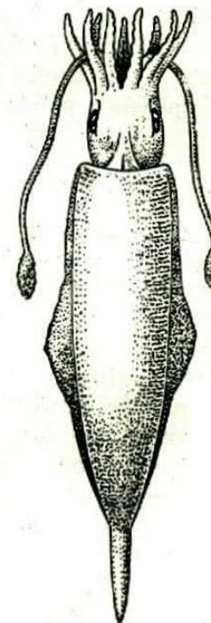
Obr. 479. Belemnites .
