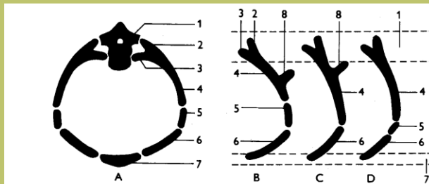
Obr. 23: Schéma organizace žebere amniot. A - hrudní segment v předozadní projekci, B - třídlínné žebro plazů, C - dvoudílné žebro ptáků, D - třídlínné žebro primátů a mravenečnicka. 1 - topografická poloha obratle, 2 - tuberculum costae, 3 - caput costae, 4 - vertebrocostale, 5 - intercostale, 6 - sternocostale, 7 - topografická poloha sternu, 8 - processus uncinatus. Upraveno podle Portmanna, 1965.
