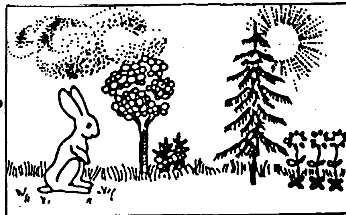
Geobiocenóza = ekosystém
