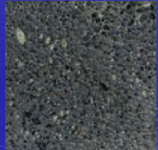
čedič bazalt
