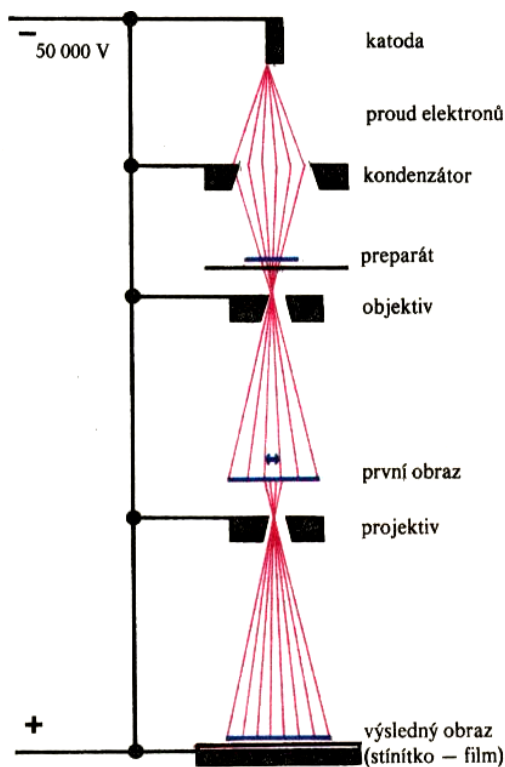
Obr.4.54. Elektronový mikroskop.
