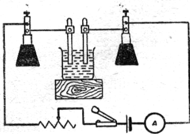
Obr.5.19. Základní zapojení pro studium vedení elektřiny v kapalinách.
