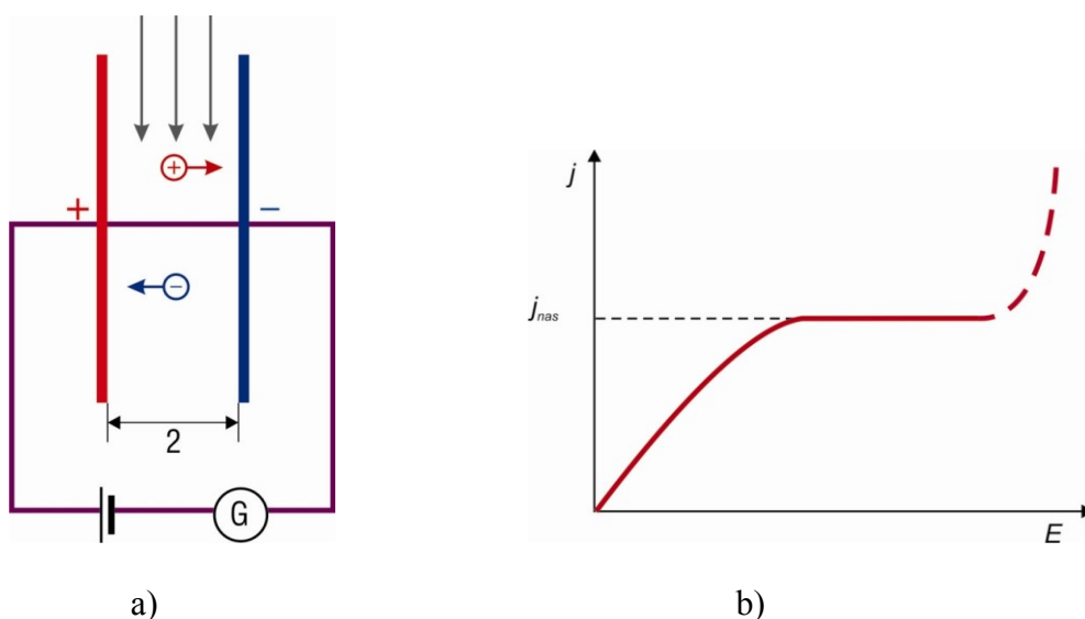
Obr.2.1 a) Schematické znázornění experimentálního uspořádání pro studium vedení elektriny v plynech. b) Voltmapérová charakteristika nesamostatného výboje v plynech.
