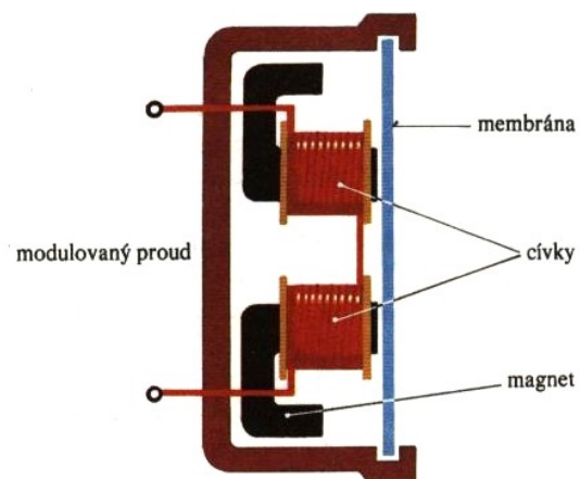
Obr.4.60. Telefonní sluchátka.
