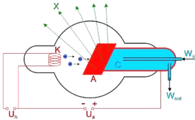
Obr2.9. Schéma rentgenky
