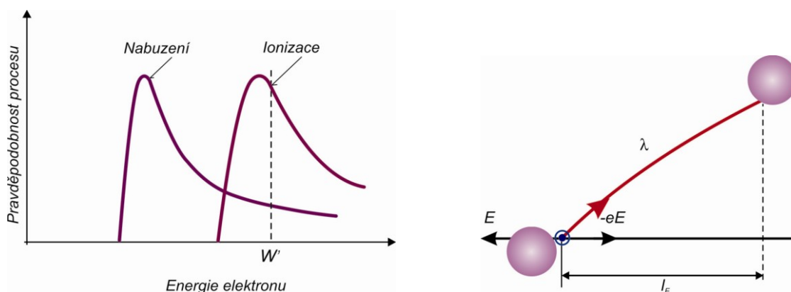
Obr.2.5a) Průběh pravděpodobnosti při nárazu molekul. b) Skutečná dráha částice v plazmatu
