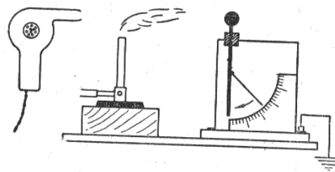
Obr.5.22. Ionizační účinky plamene.
