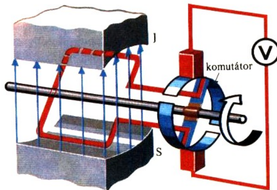
Obr.4.16. Dynamo.
