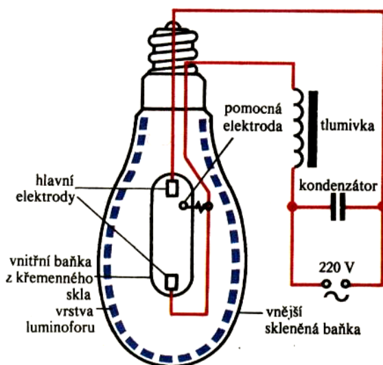
Obr.4.44. Rtuťová výbojka.
