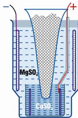
Obr.1.7b) Meidingerův článek
