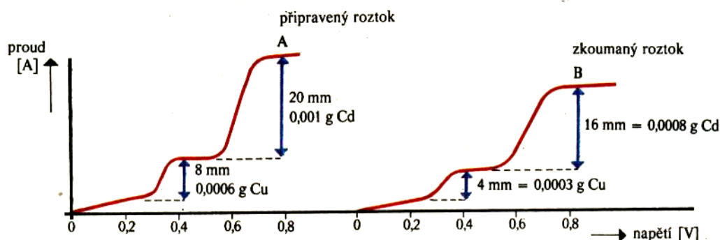
Obr.4.28b) Kvantitativní polarografie.
